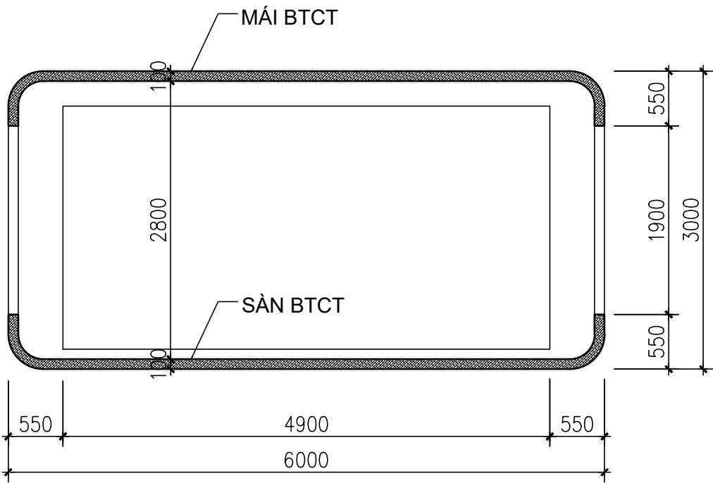
MẶT CẮT DỌC
