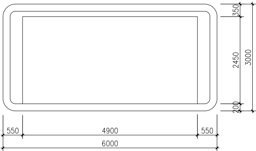
MẶT ĐỨNG TRƯỚC
